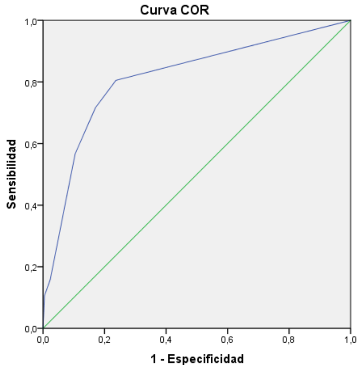
Fig. 2 - Curva ROC de variables cardiovasculares y mortalidad.
